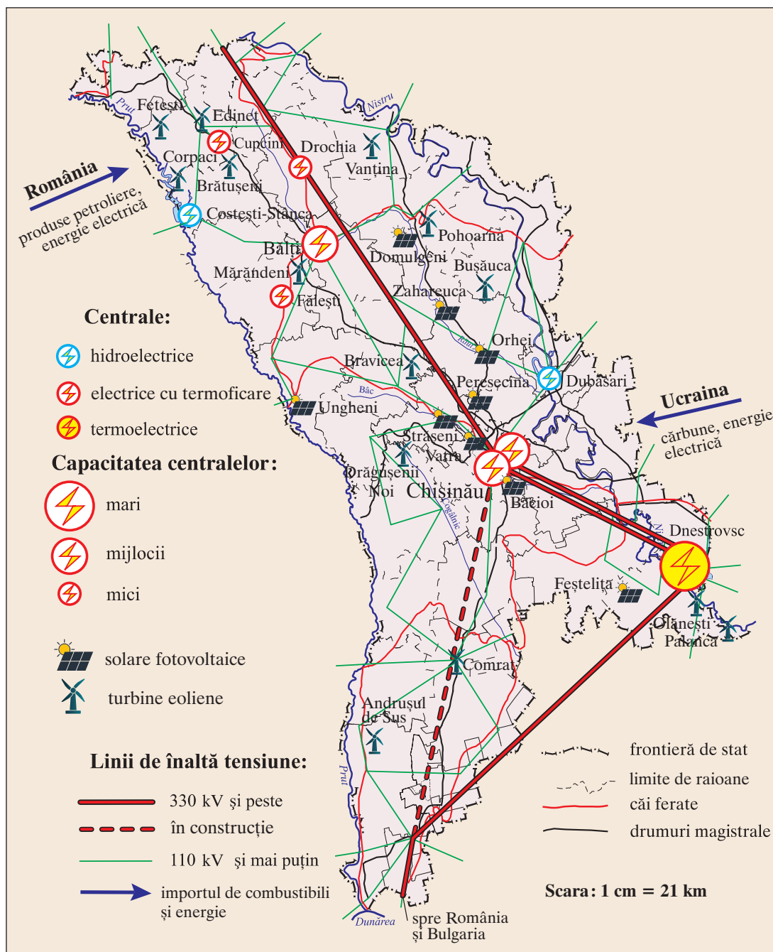
Fig. 3.43. Industria energetică
