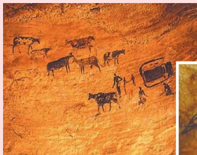
Picturi rupestre din grota de la Coliboaia, județul Bihor (circa 35.000 de ani în urmă)
